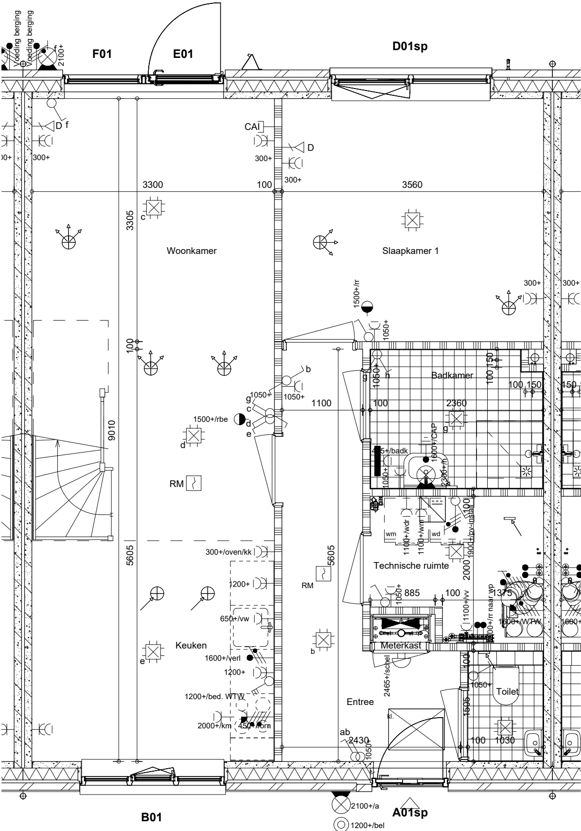
begane grond
