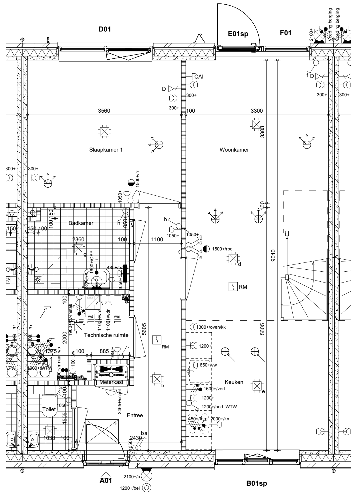
begane grond
