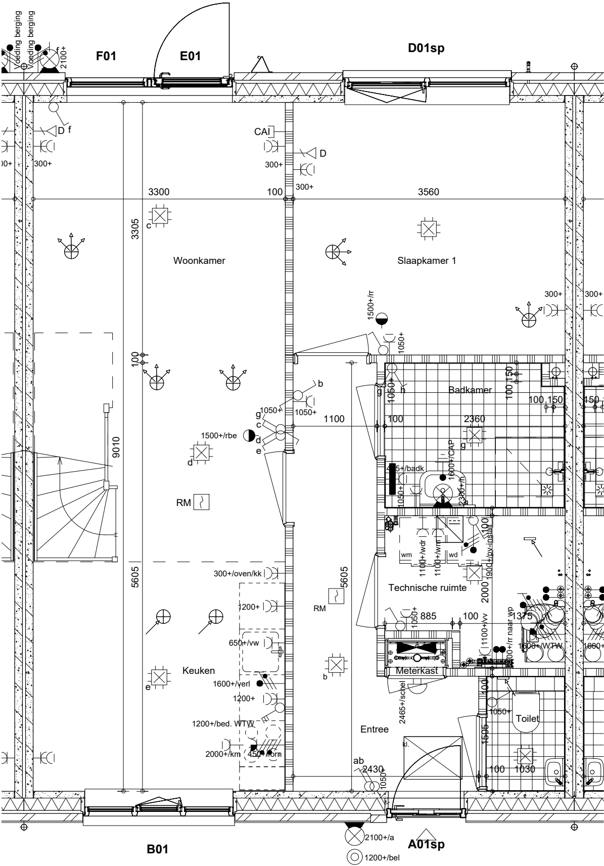
begane grond
