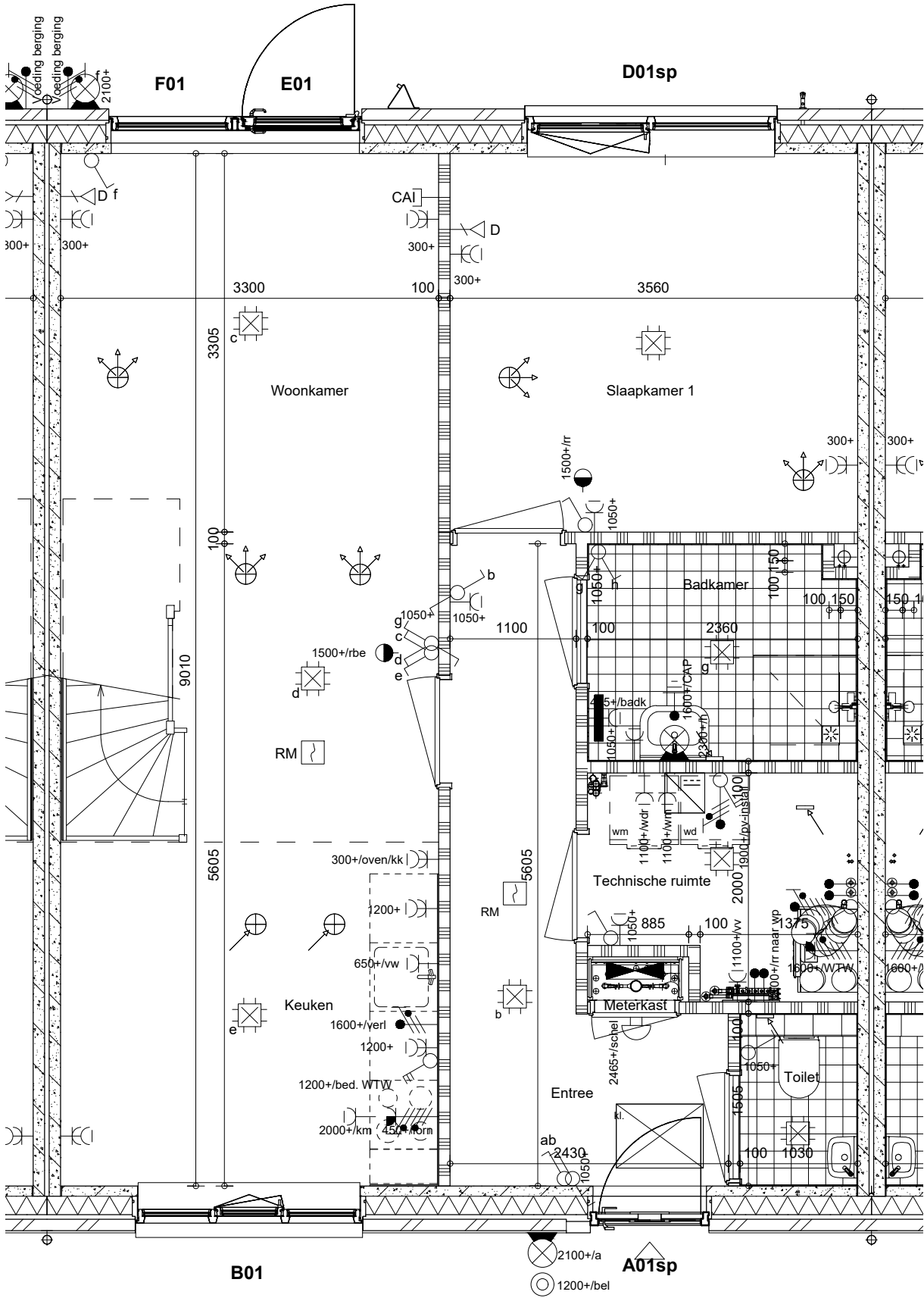
begane grond
