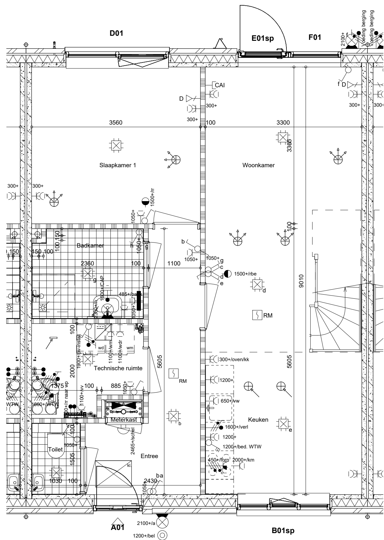
begane grond
