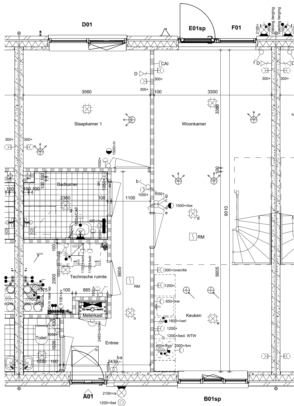
begane grond
