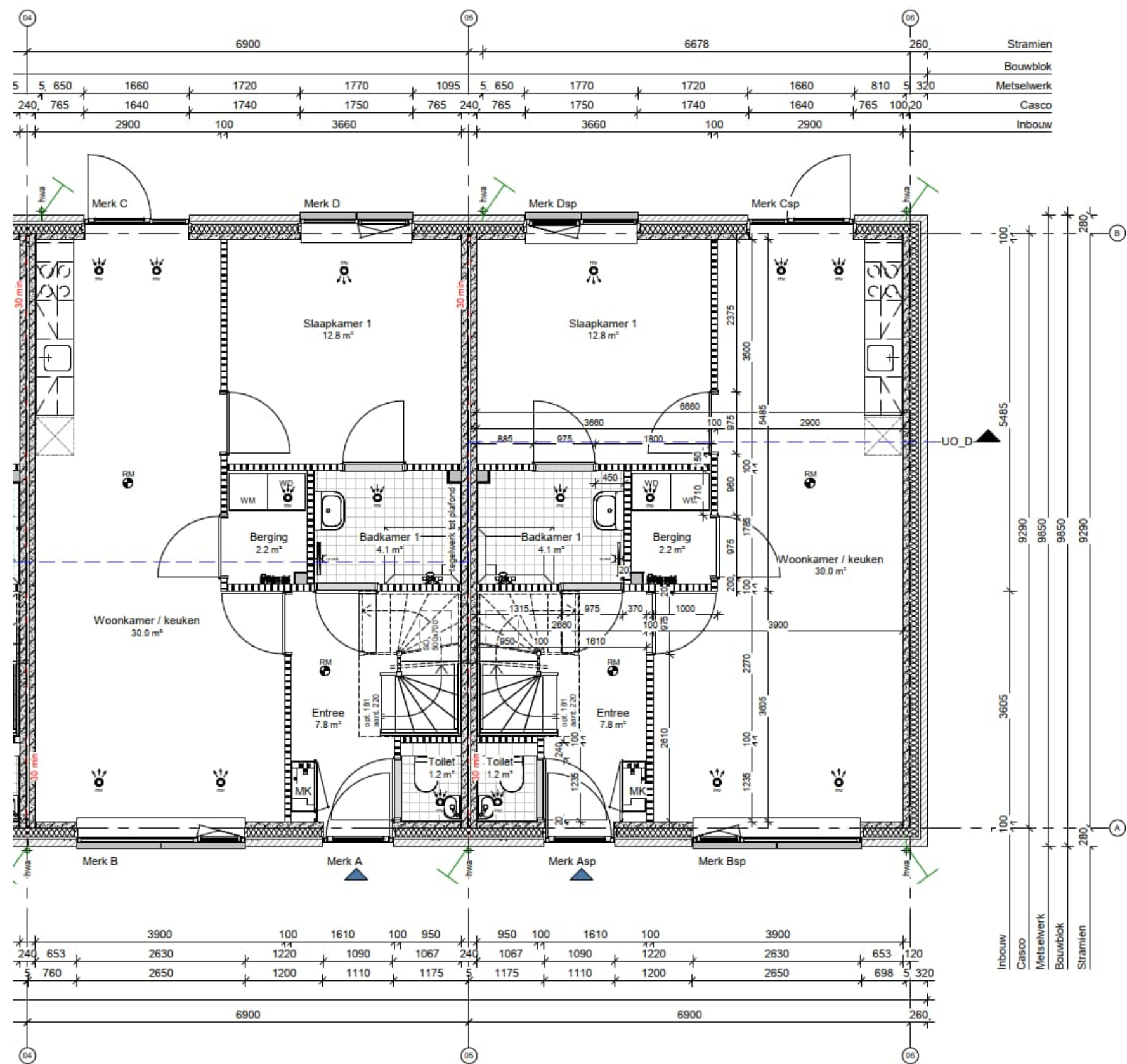
Getekende woning
