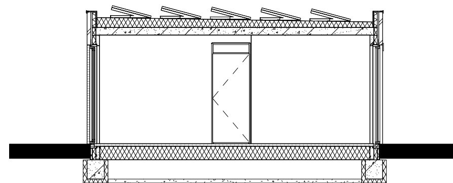
doorsnede Henri Dunantstraat 9 en 11
