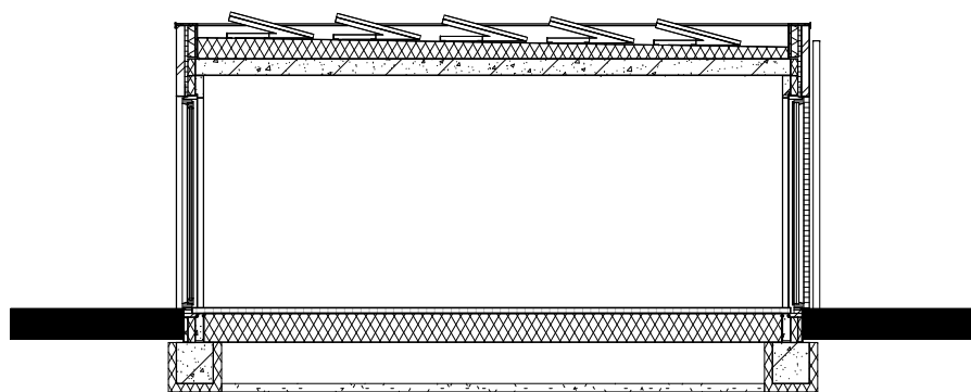
doorsnede Henri Dunantstraat 7
