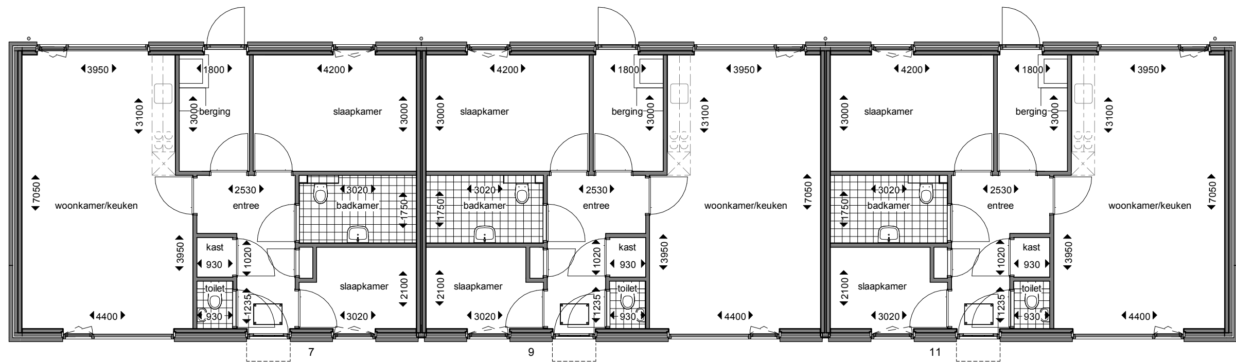
begane grond Henri Dunantstraat 7 t/m 11
